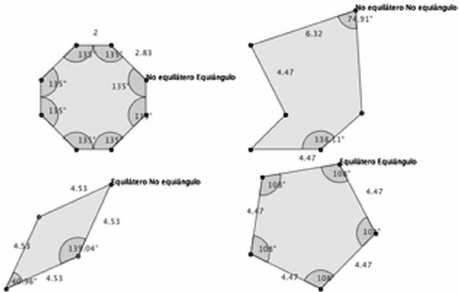
Figura 20. Equiángulo y / o equilátero
