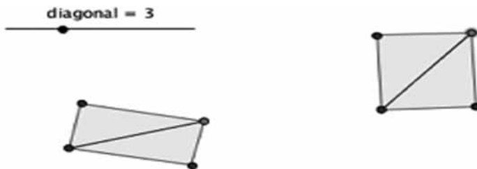
Figura 21. Cuadrilátero de diagonal dada
